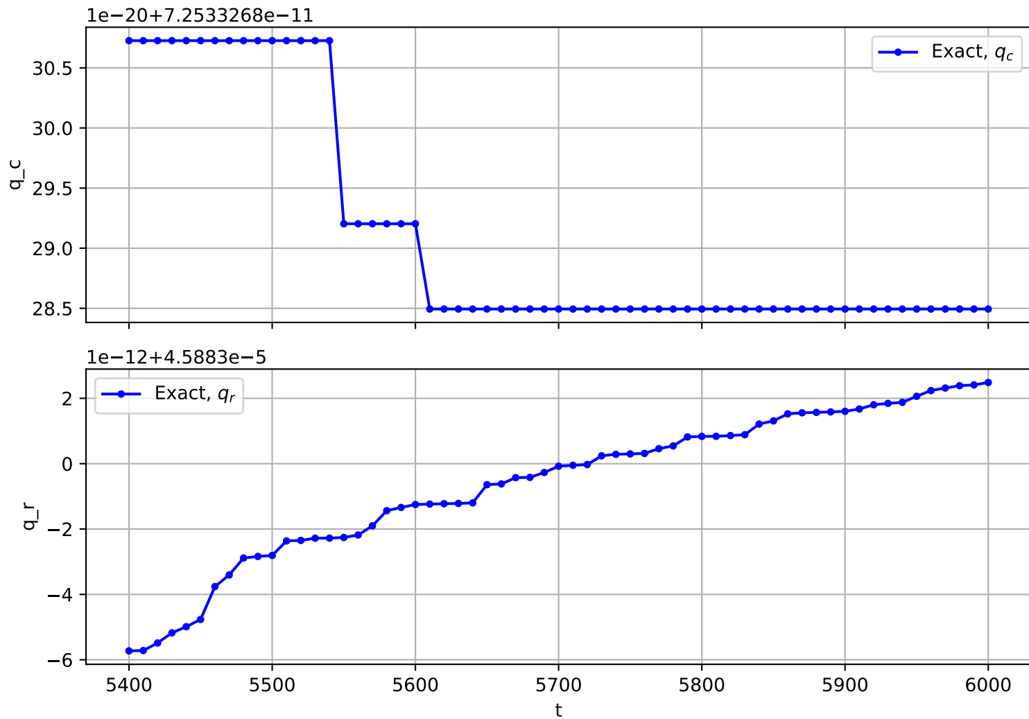
Trajectory No. 3437
