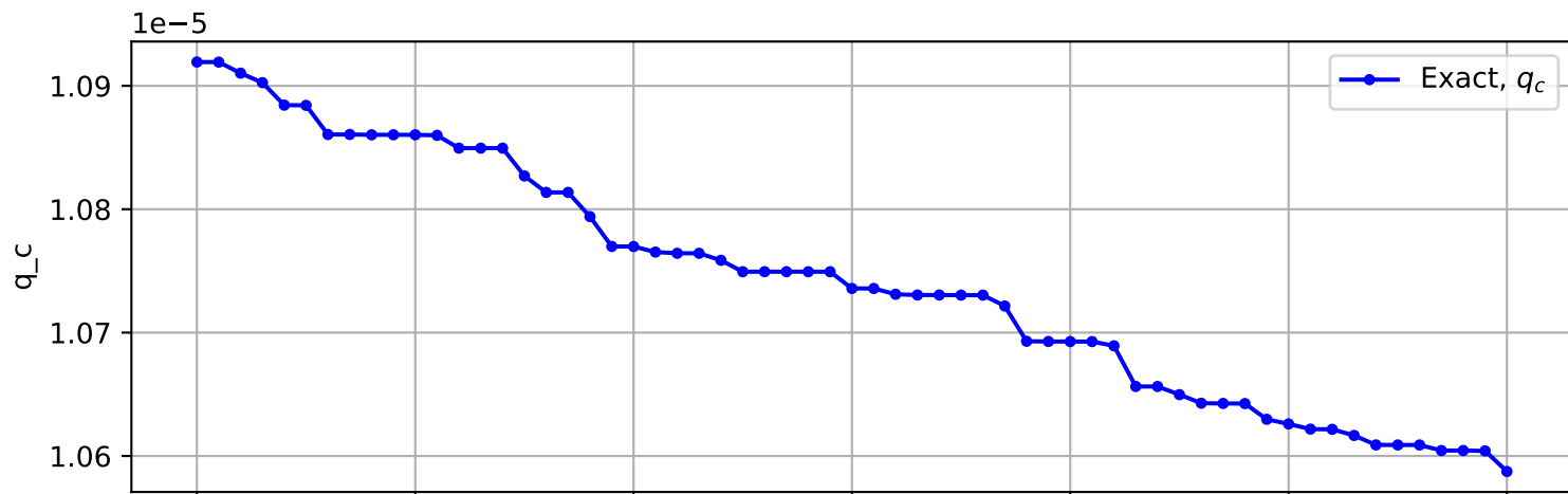
Trajectory No. 3443
