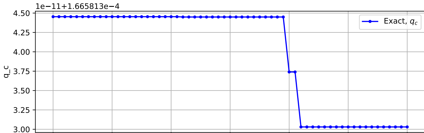
Trajectory No. 3448
