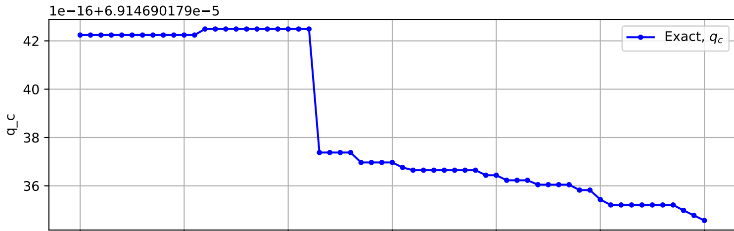
Trajectory No. 3454
