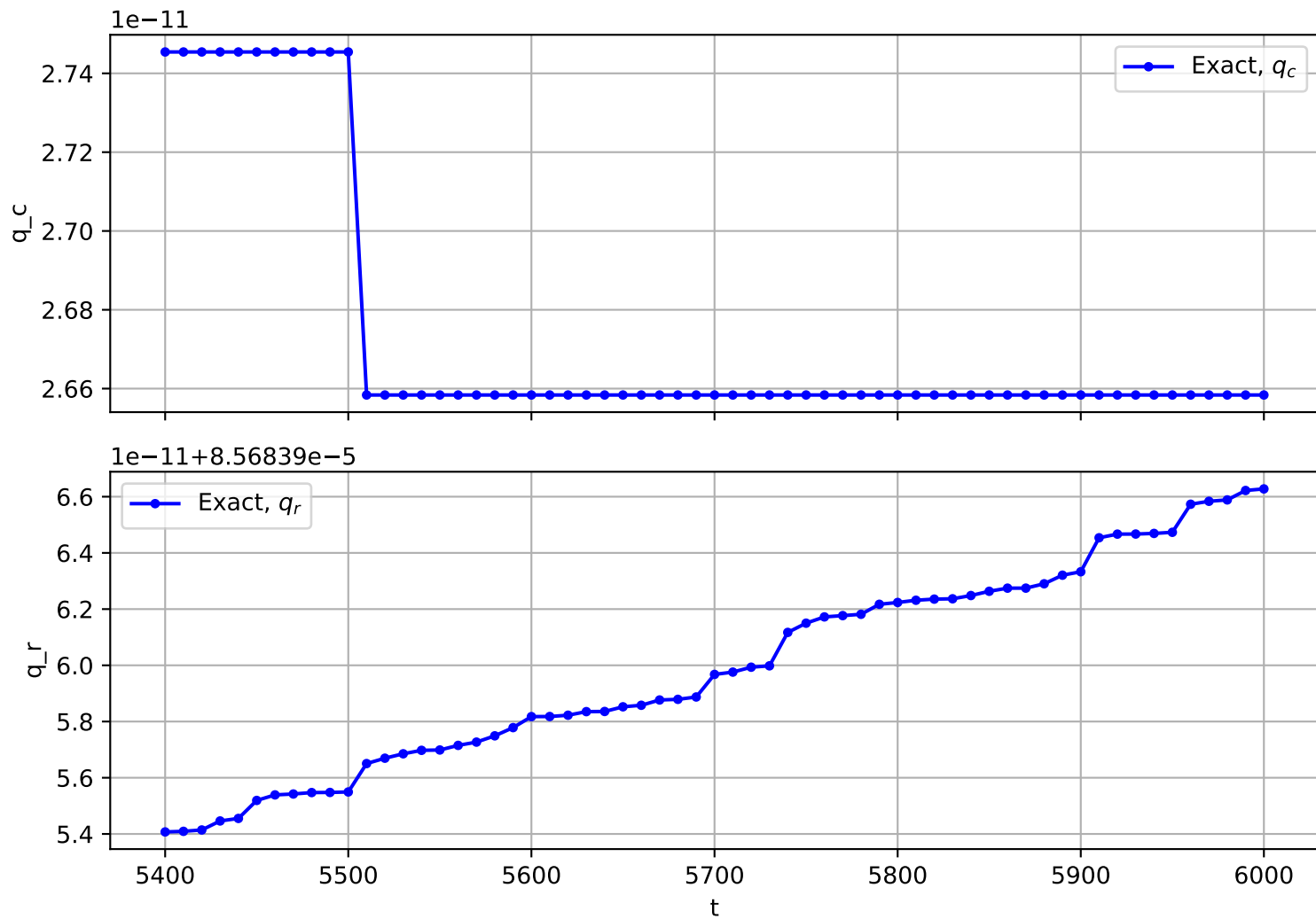
Trajectory No. 3477
