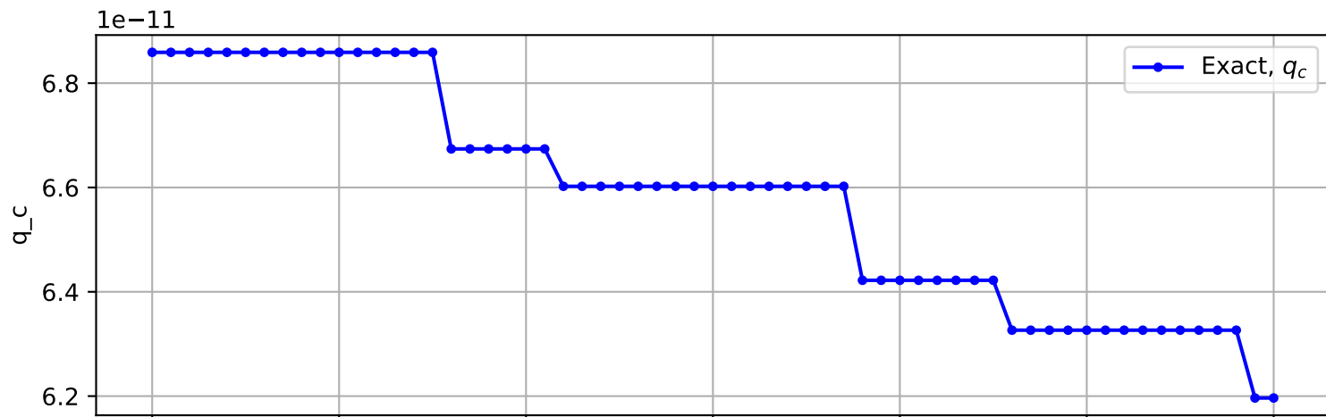
Trajectory No. 3495
