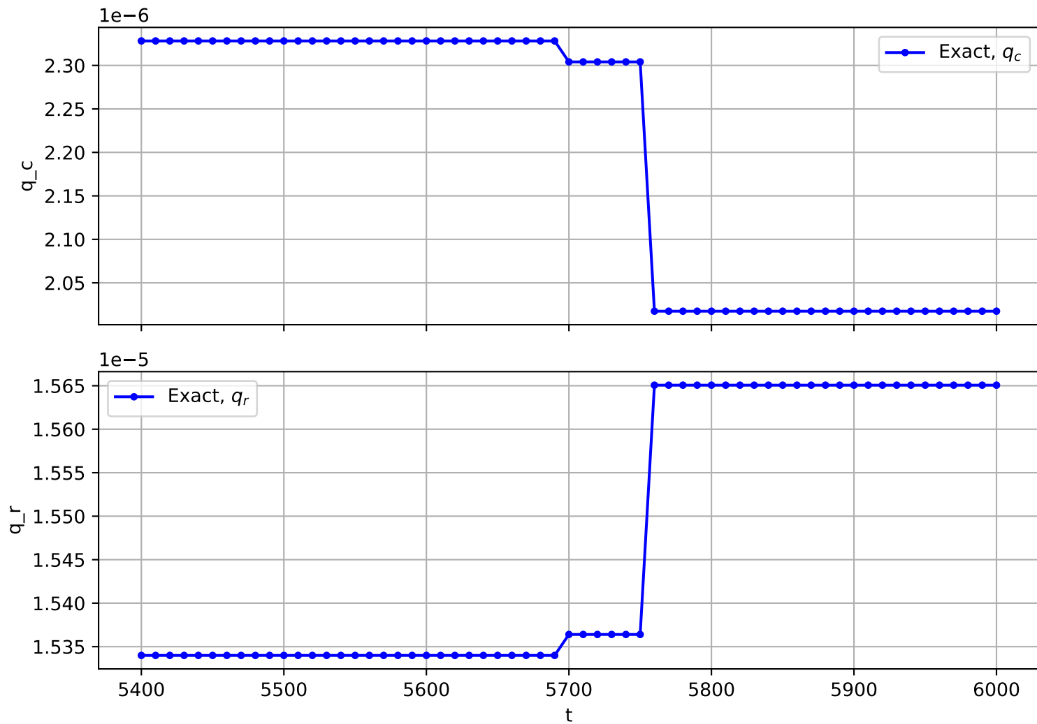
Trajectory No. 3512
