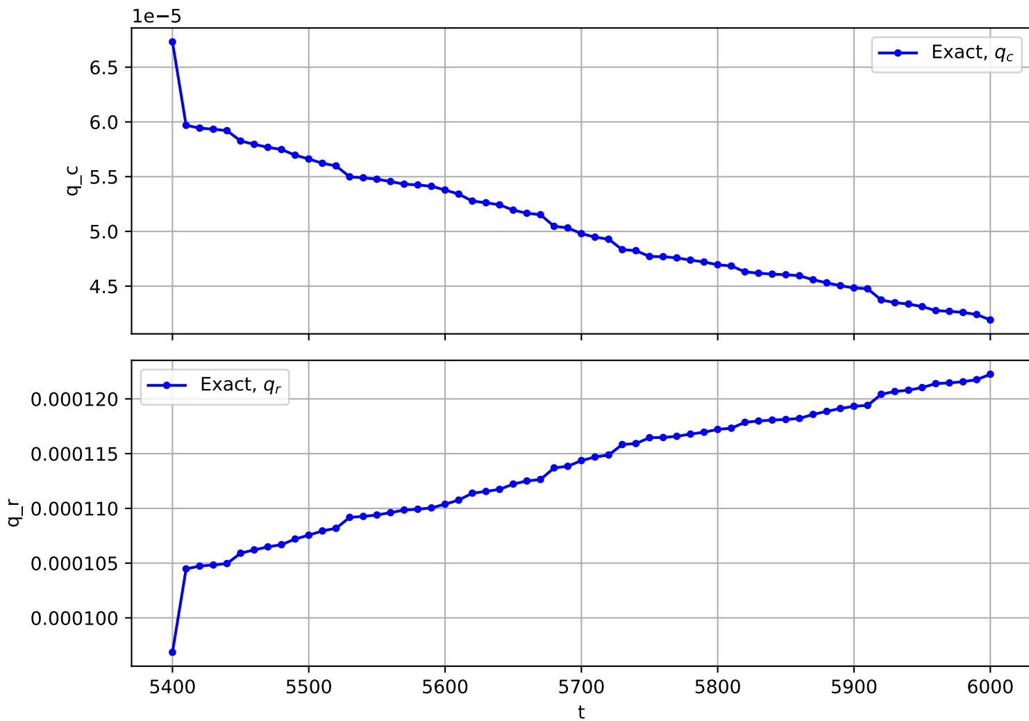
Trajectory No. 382
