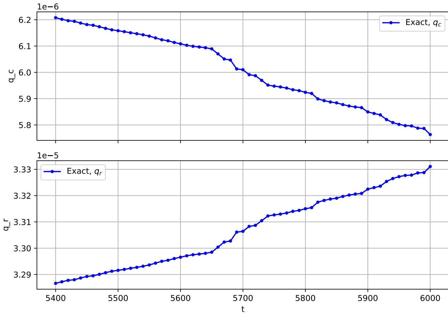
Trajectory No. 461
