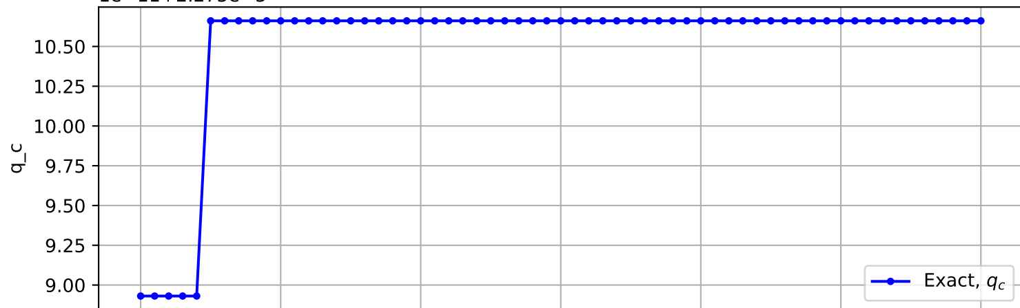
Trajectory No. 492
