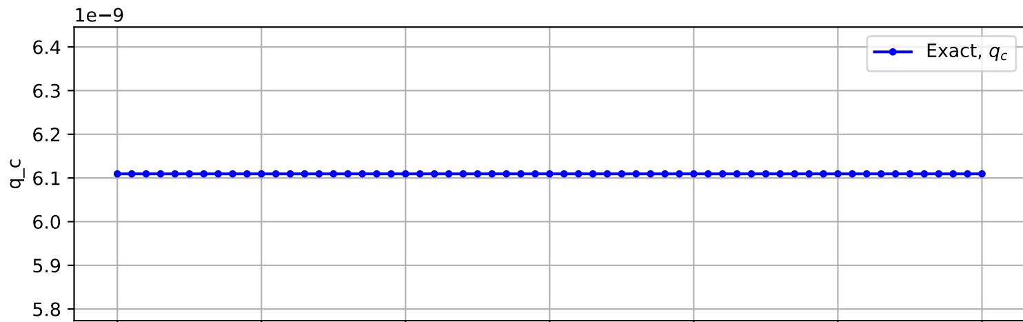
Trajectory No. 564
