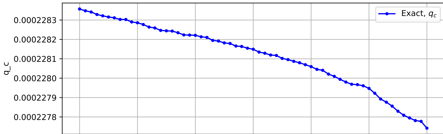
Trajectory No. 596
