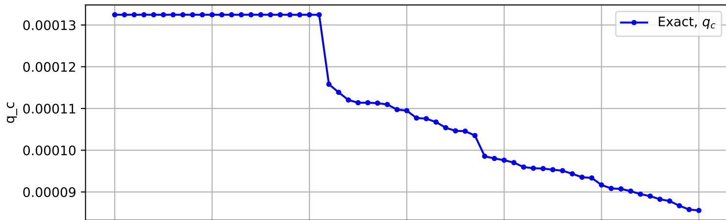
Trajectory No. 616
