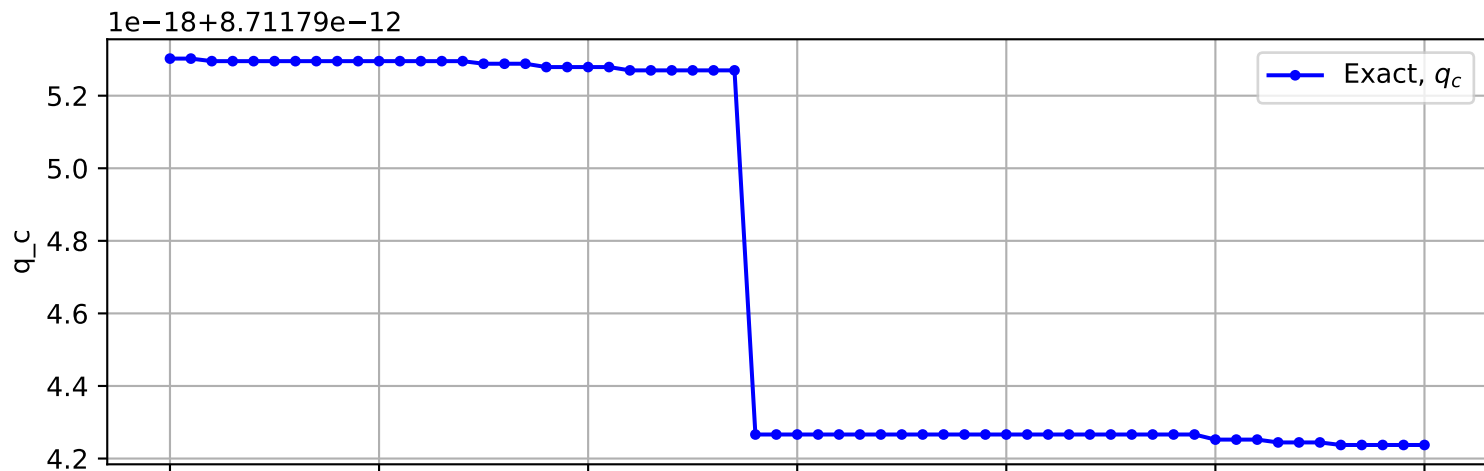
Trajectory No. 720
