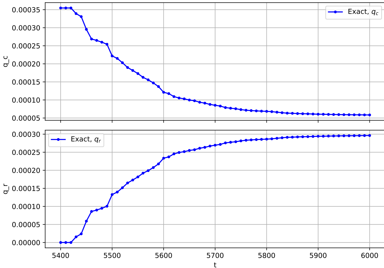
Trajectory No. 780
