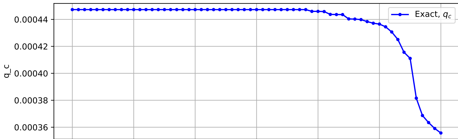
Trajectory No. 791
