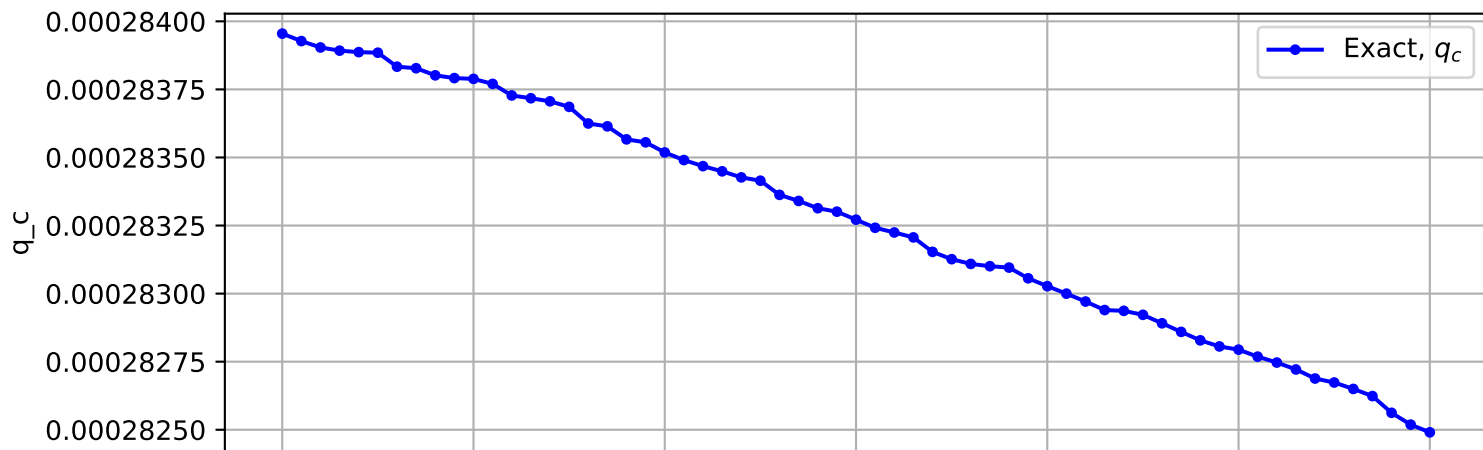
Trajectory No. 821
