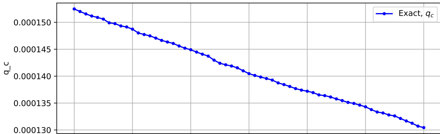
Trajectory No. 831
