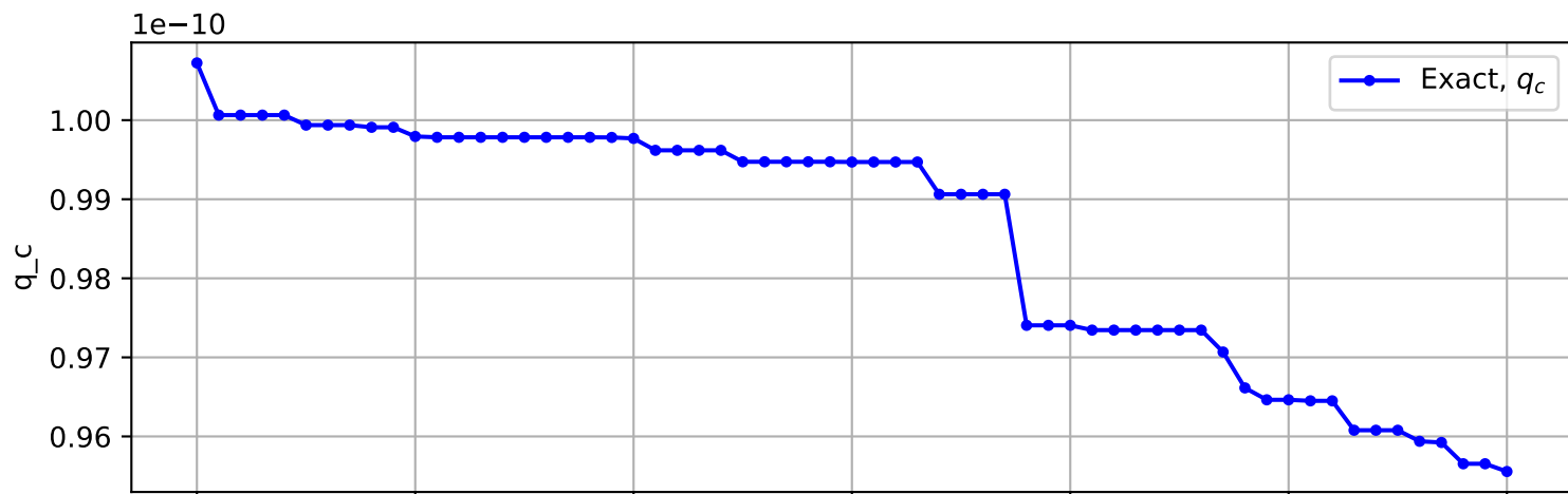
Trajectory No. 884
