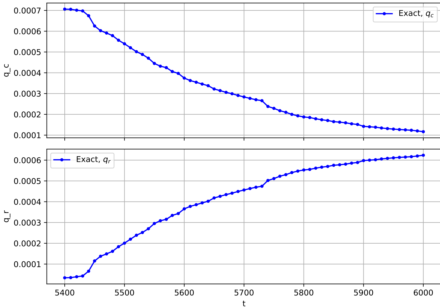
Trajectory No. 891
