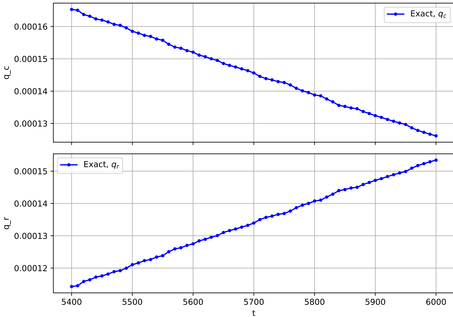
Trajectory No. 917
