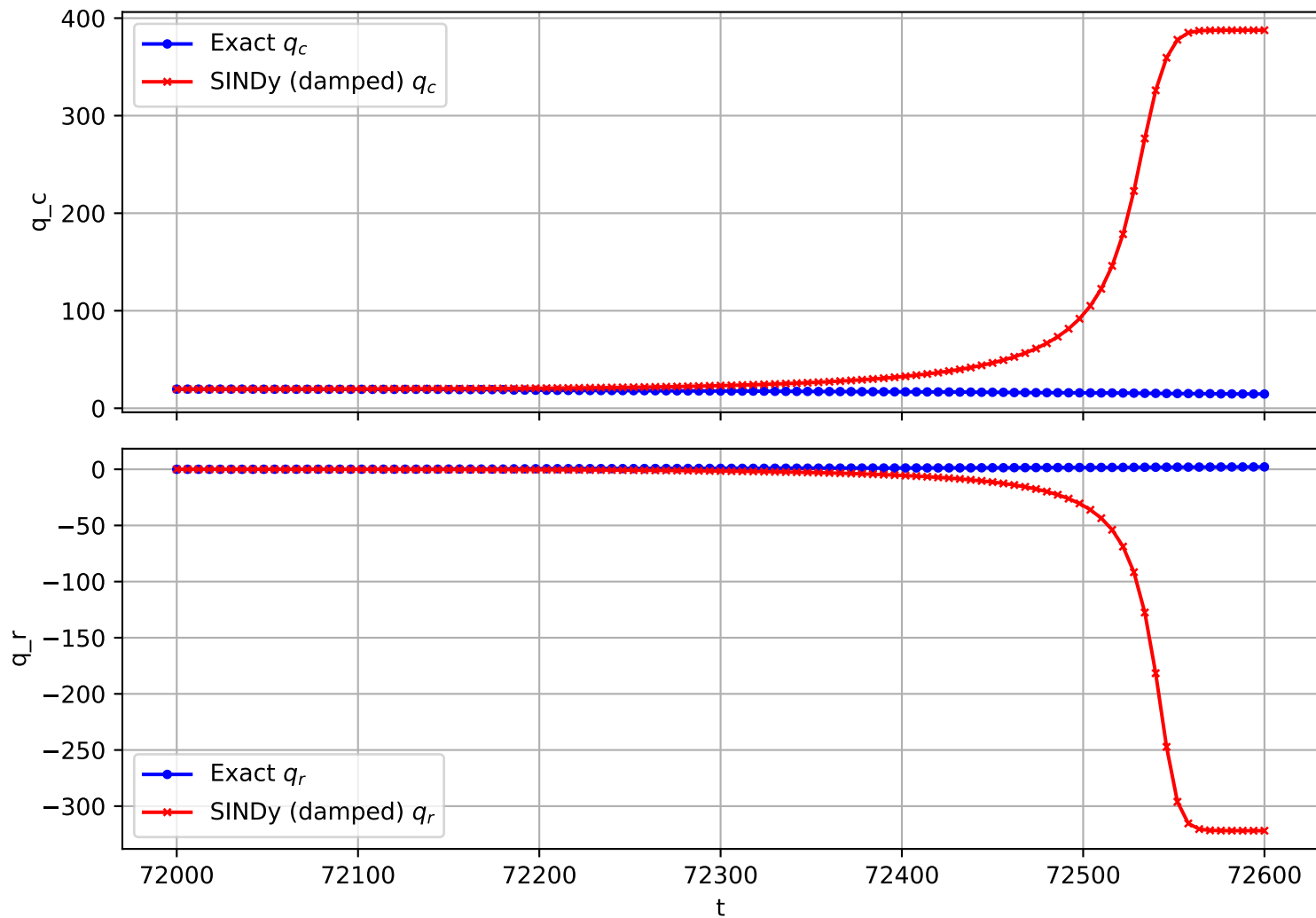
Trajectory 165 (damped)
