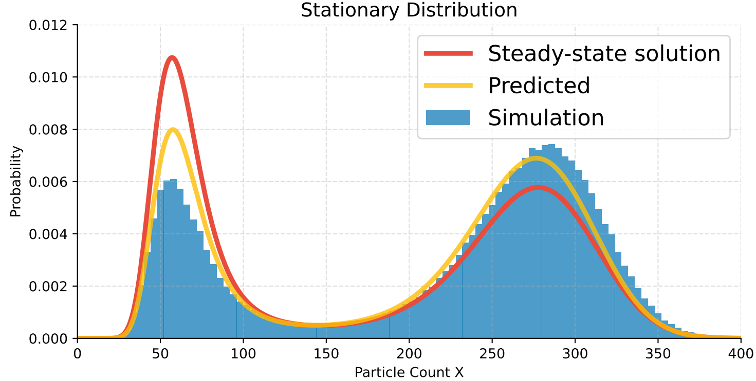
(d) Case 4: \gamma = 0.5477, D = 750, \tau = 1 \times 10^{-6}
