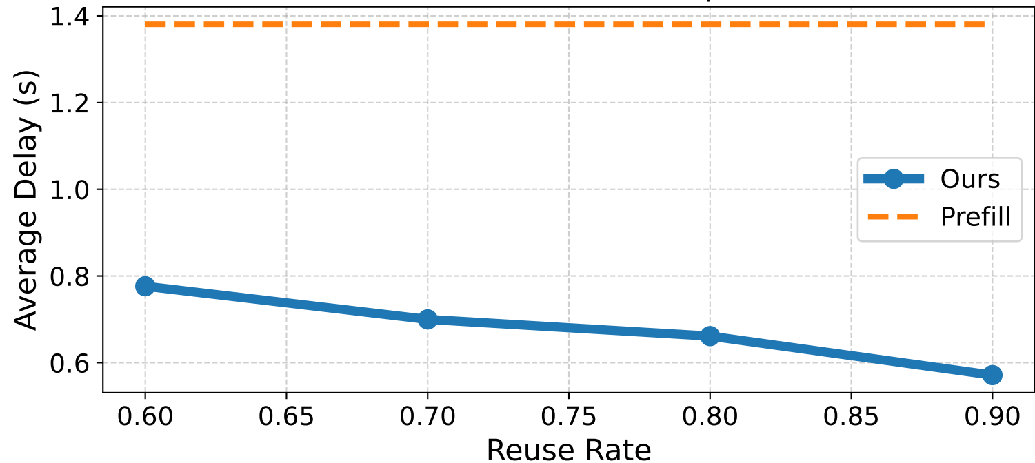
Min TTFT for F1 Score Drop < 5%
