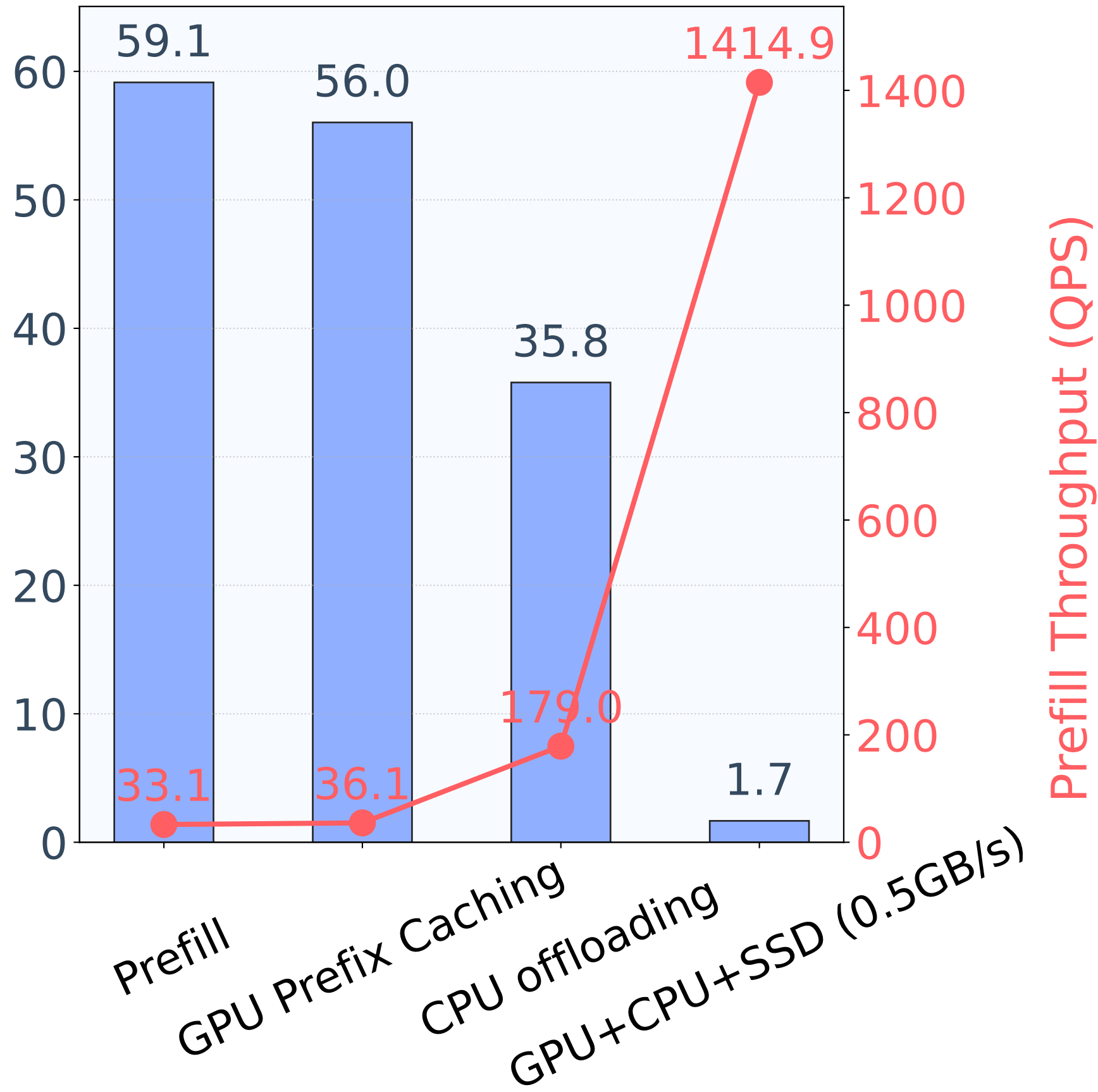
Llama-3.1-8B
