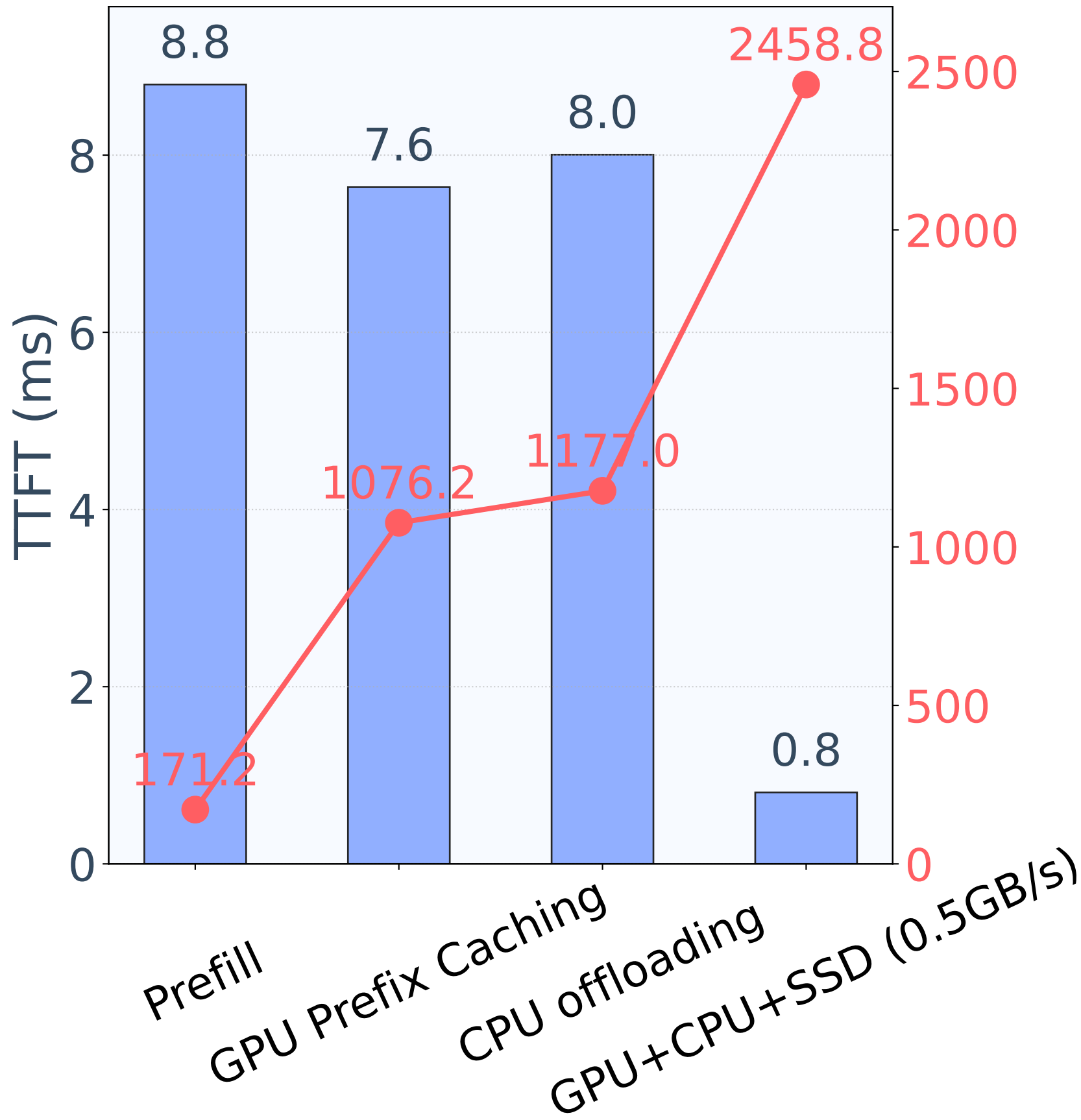
Llama-3.2-3B
