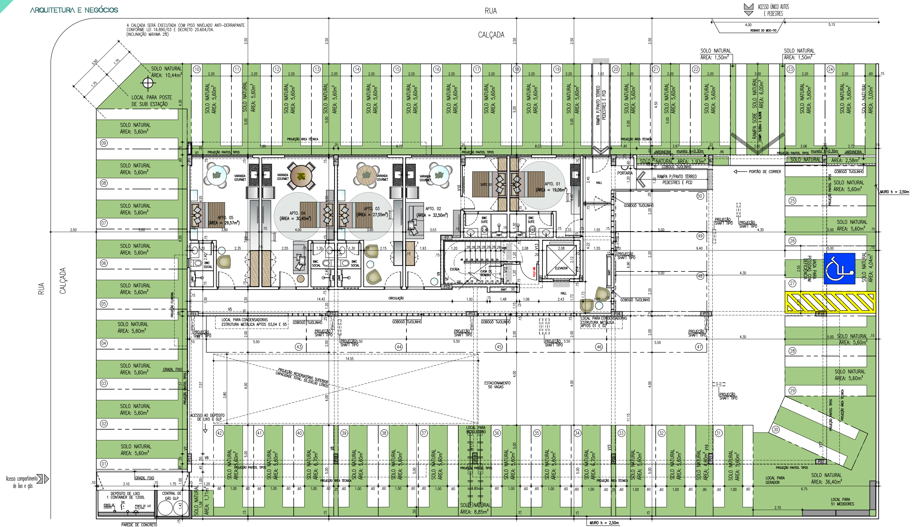
PLANTA BAIXA – TÉRREO ESCALA: S/E
