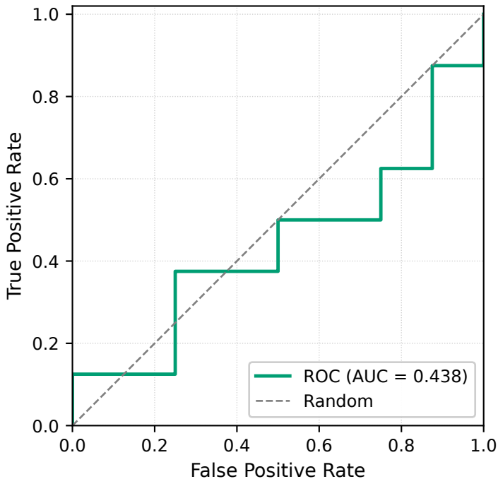
data1 — CatBoost (n=16)
