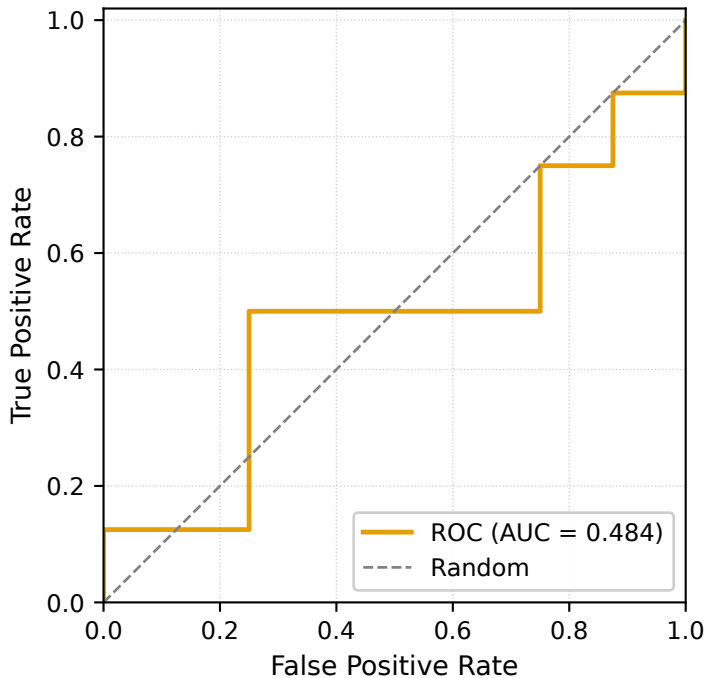
data1 — XGBoost (n=16)
