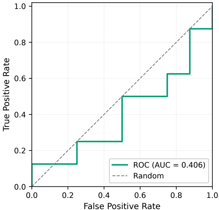
data2 — CatBoost (n=16)
