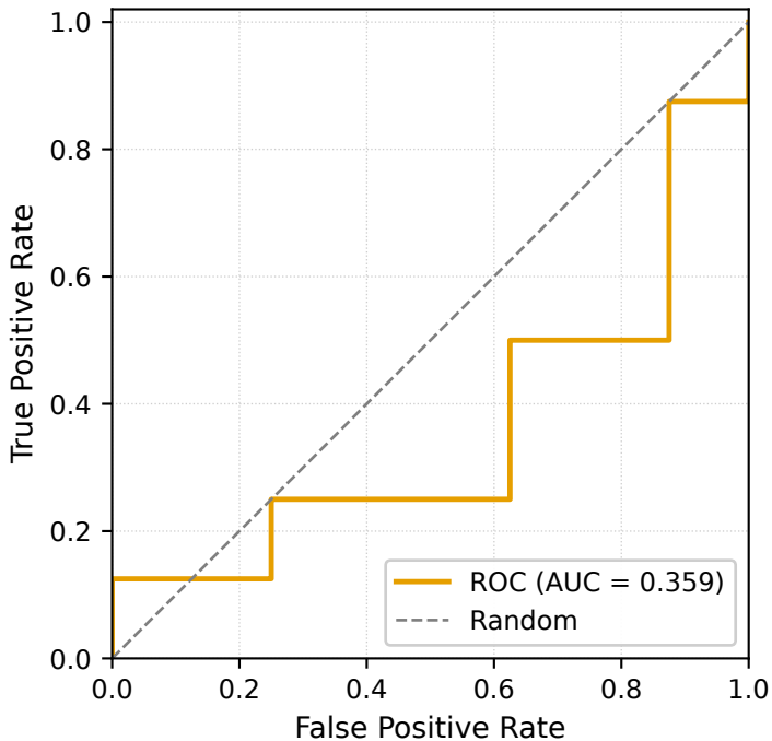
data2 — XGBoost (n=16)
