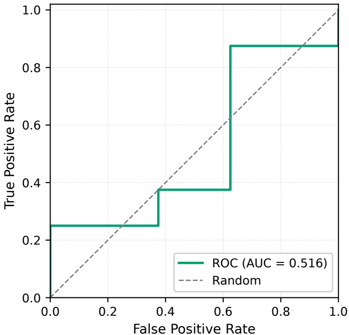
data3 — CatBoost (n=16)
