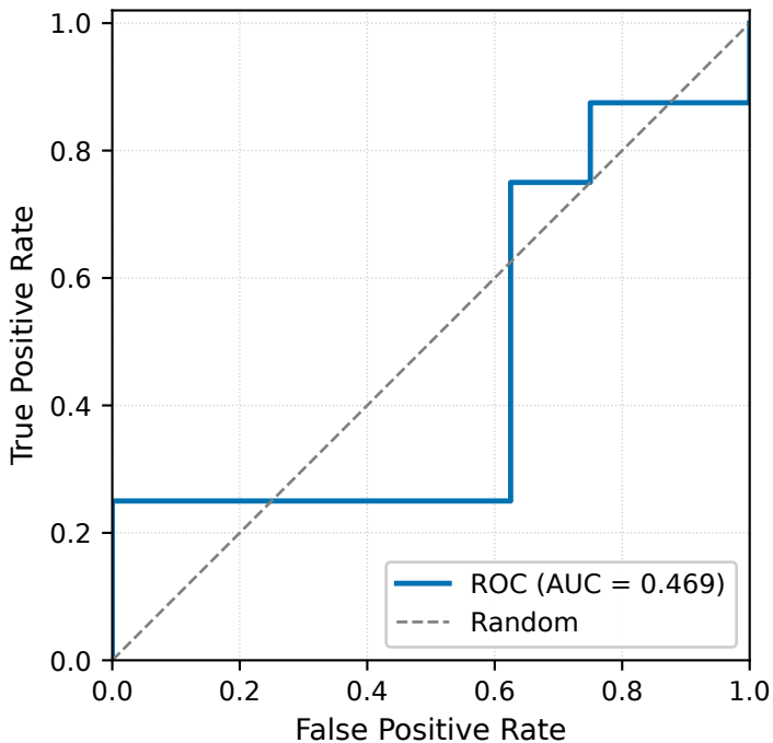
data3 — LightGBM (n=16)
