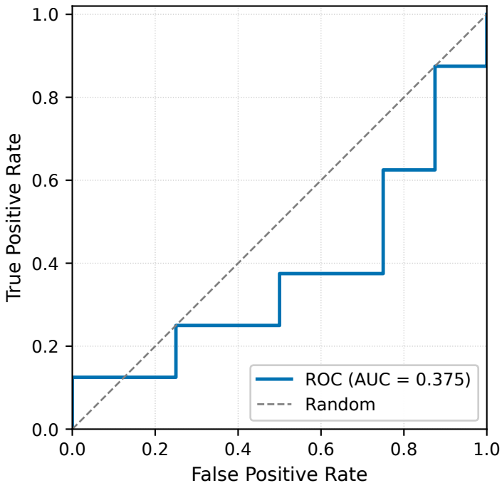
data2 — fold 1 (n=16)
