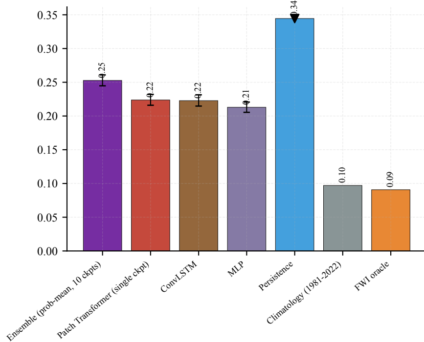
PR-AUC
