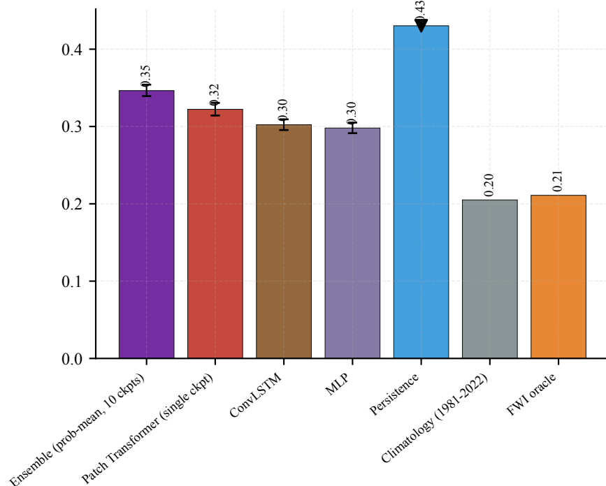
PR-AUC
