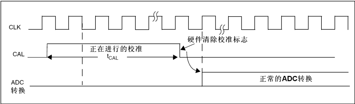
图28 校准时序图
