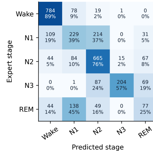
A6 ensemble Acc 0.651 · F1 0.586
