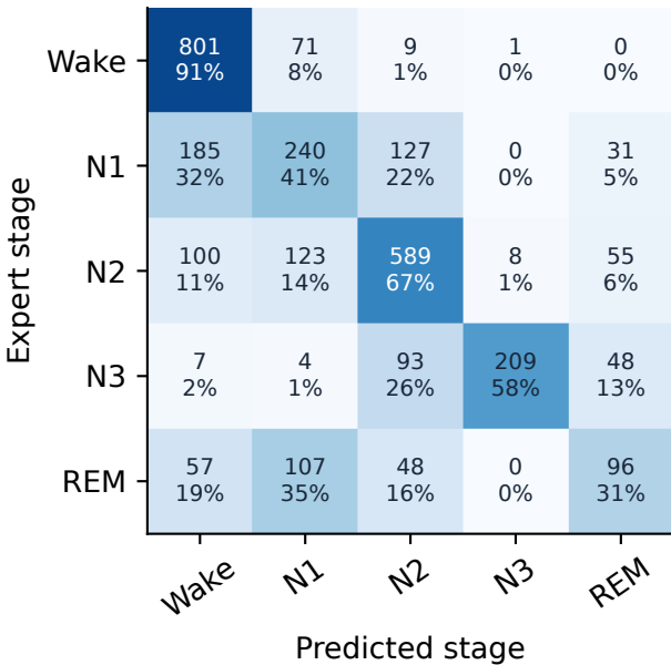
A4 ensemble Acc 0.643 · F1 0.594
