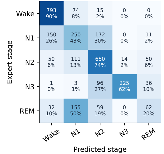
A3 ensemble Acc 0.658 · F1 0.594
