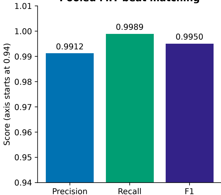
Pooled MIT beat matching
