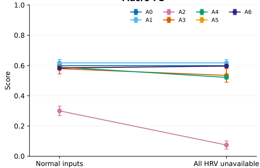
Macro-F1
