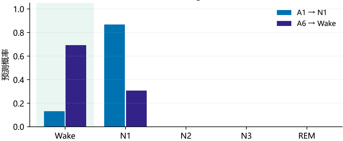
仅 A6 正确 • ISRUC-III-04 / epoch 27 专家: Wake • A6 gate=0.218
