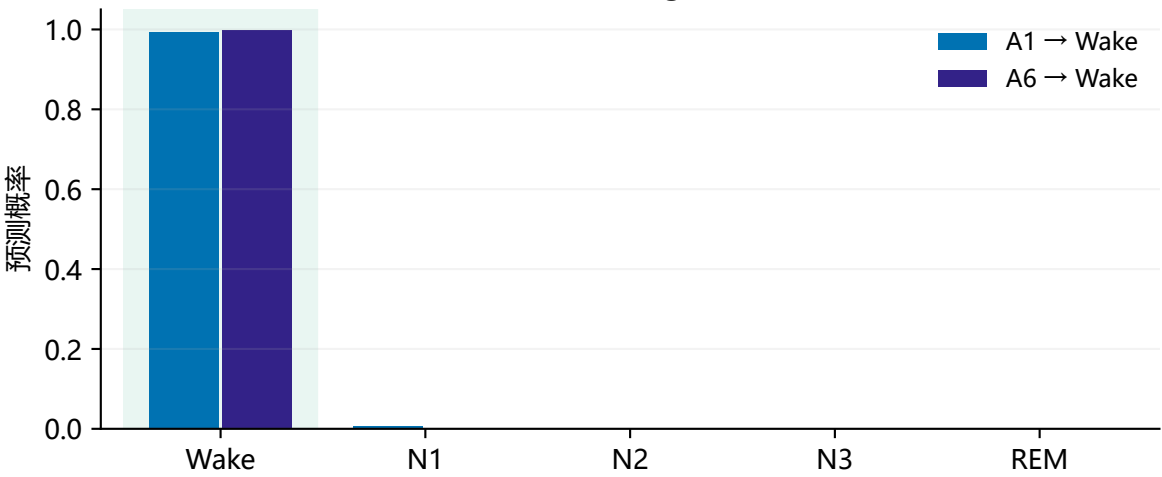
两者正确 • ISRUC-III-04 / epoch 14 专家: Wake • A6 gate=0.301
