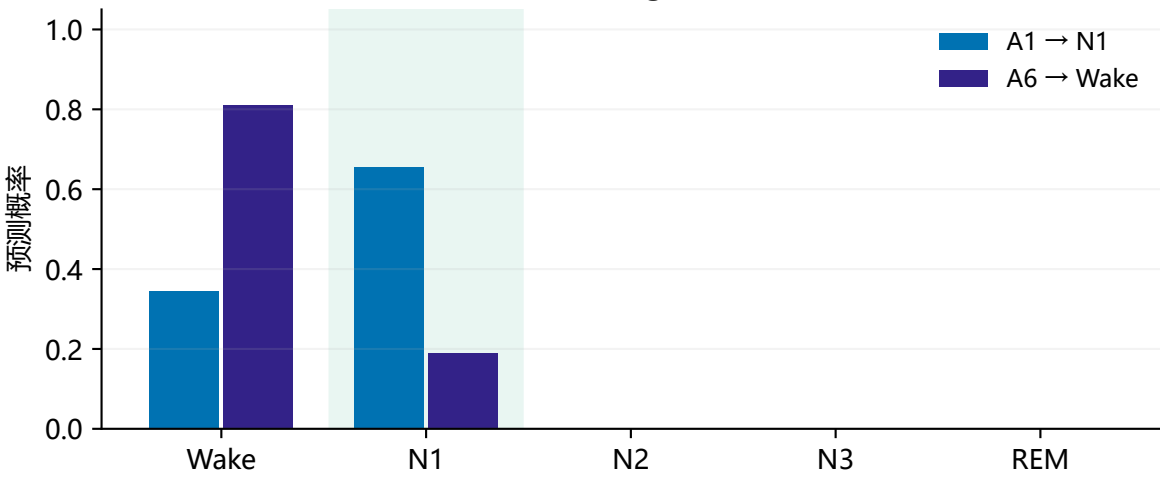
仅 A1 正确 • ISRUC-III-04 / epoch 29 专家: N1 • A6 gate=0.198
