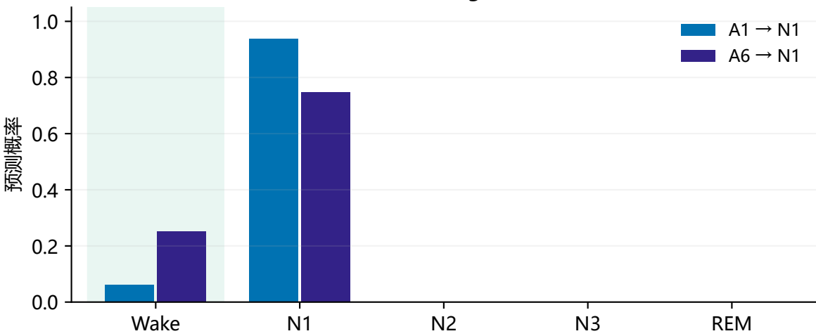
两者错误 • ISRUC-III-04 / epoch 26 专家: Wake • A6 gate=0.333
