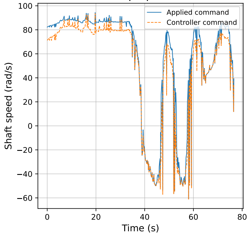
Left propeller
