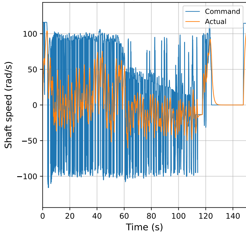
Left propeller
