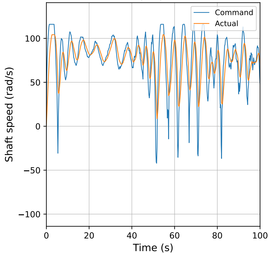
Left propeller
