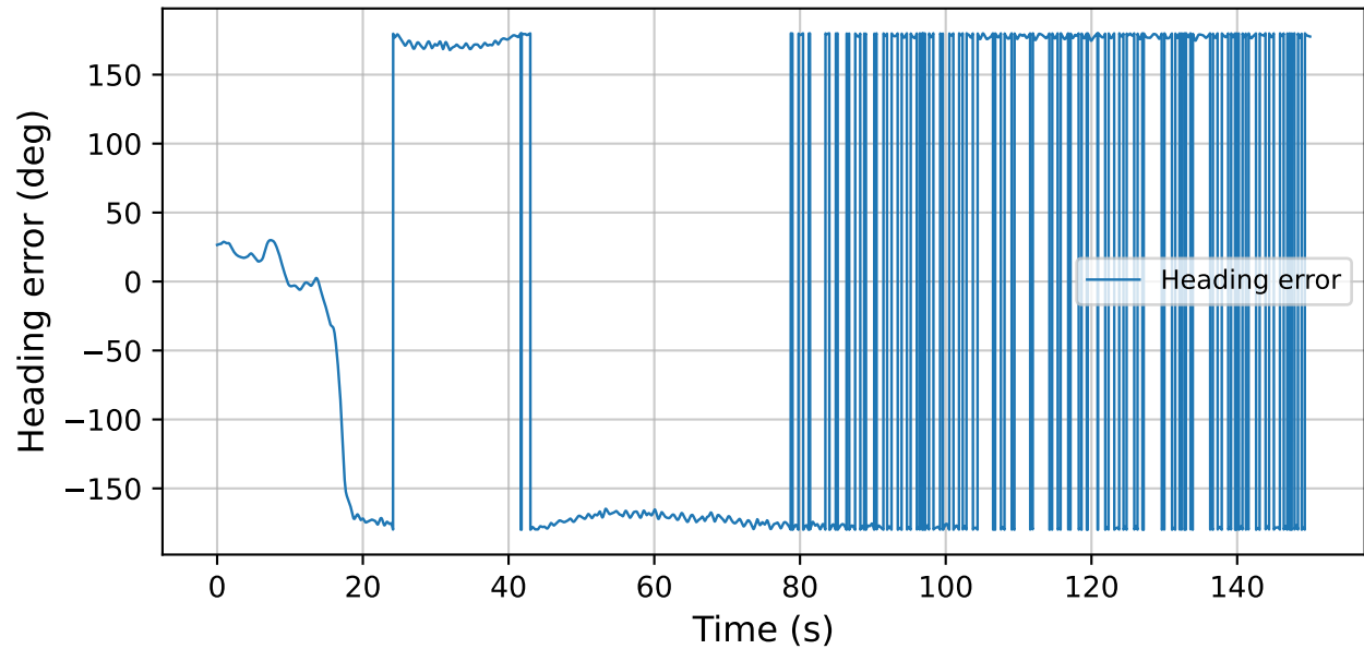
NMPC heading error
