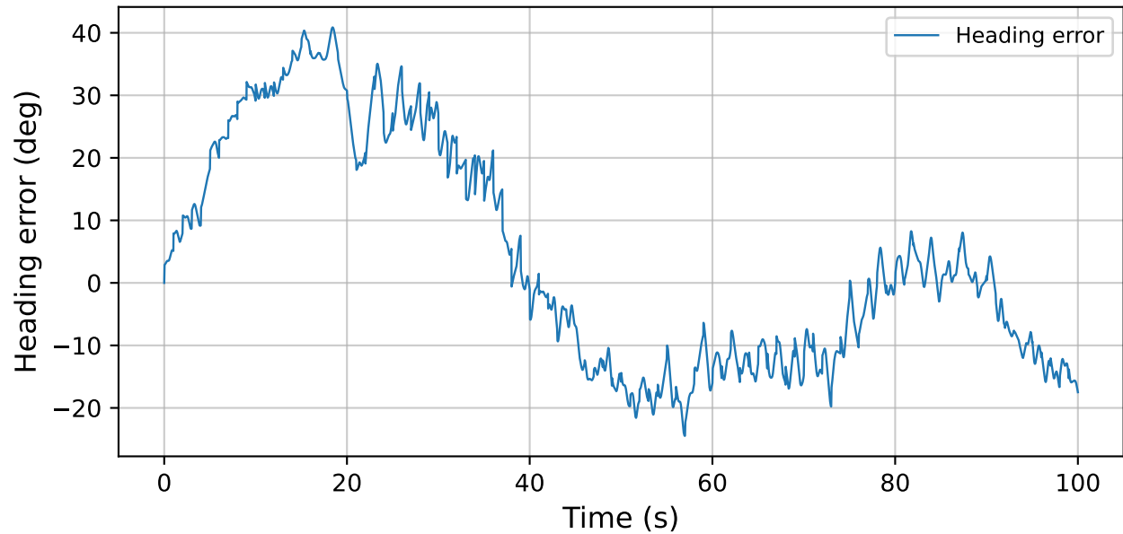
PID heading error
