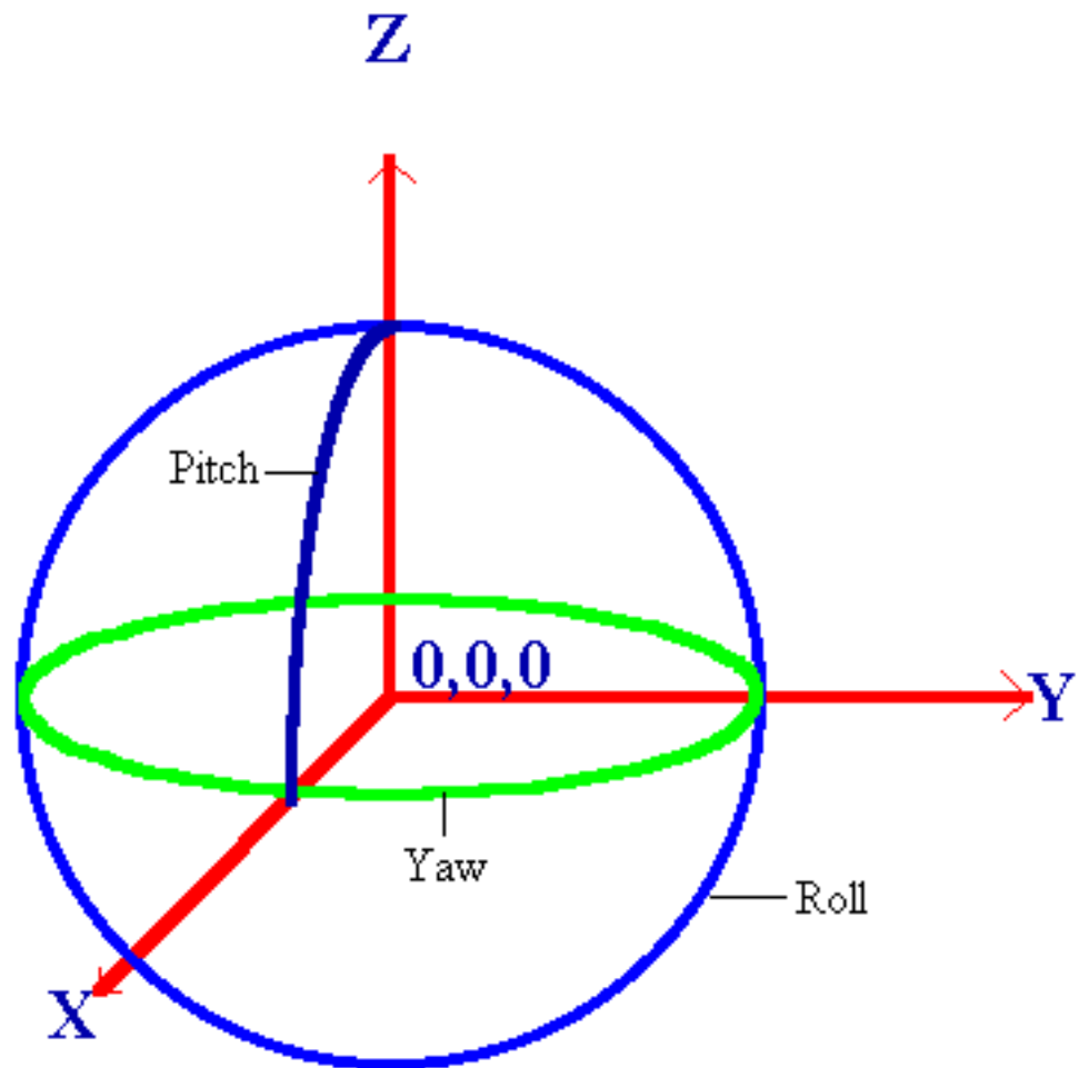
Abbildung 19: Euler-Winkel-System - Quelle: https://www.researchgate.net/figure/yz-and-pitch-roll-and-yaw-systems_fig4_253569466 abgerufen 17.03.2026
