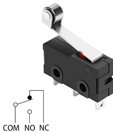
Abbildung 17: Microschalter des Wagenhebers
