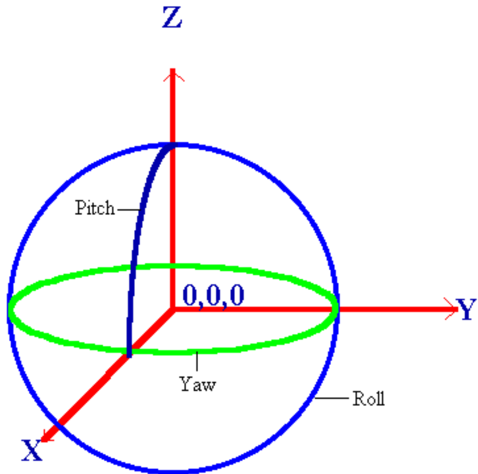
Abbildung 20: Euler-Winkel-System - Quelle: https://www.researchgate.net/figure/yz-and-pitch-roll-and-yaw-systems_fig4_253569466 abgerufen 17.03.2026
