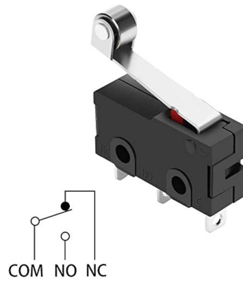
Abbildung 20: Microschalter des Wagenhebers
