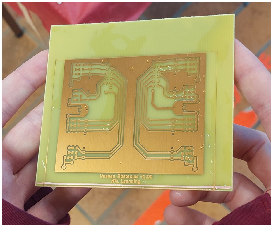
Abbildung 10: Platine Prototyp
