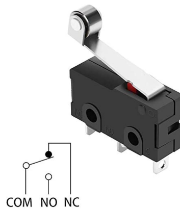
Abbildung 23: Microschalter des Wagenhebers
