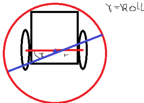
Abbildung 29: Mover hinten Berechnung - Sketch 09.01.2026
