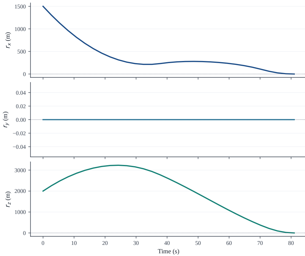
图 3 位置分量时间曲线。上: r_x ; 中: r_y ; 下: r_z 。
