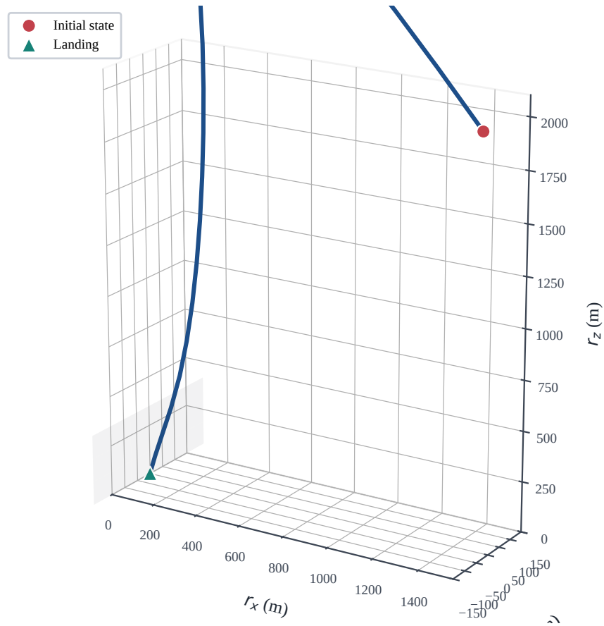
图 2 三维着陆轨迹。起始于 (1500, 0, 2000) m，终止于原点。
