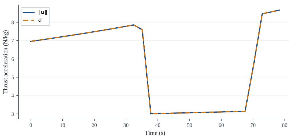
图 6 推力幅值 \|u\| 与松弛变量 \sigma 的对比。两者重合验证了无损凸化的松弛间隙为零。
