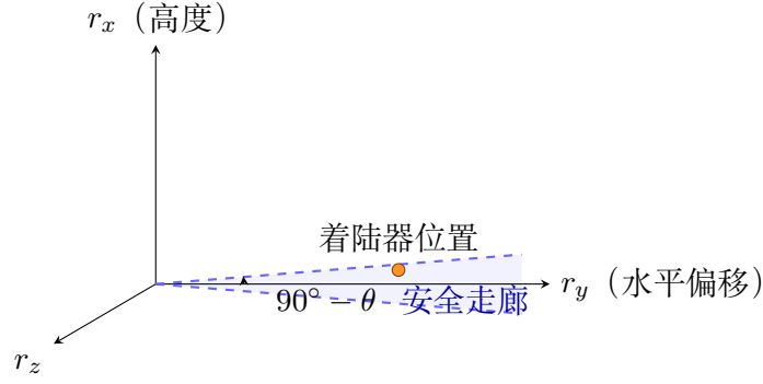
图 1 下滑角约束的几何示意图
