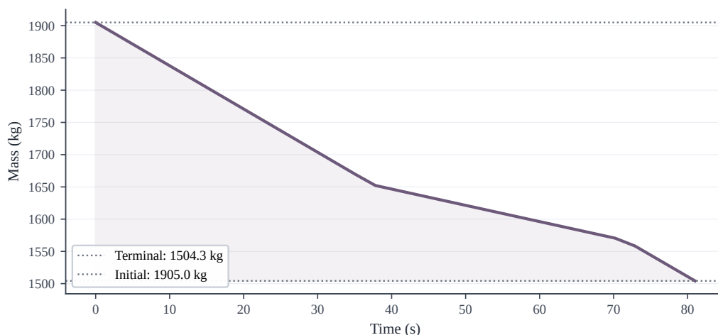
图 5 着陆器质量变化曲线。初始 1905.0 kg，终端 1504.3 kg，燃料消耗 400.7 kg。
