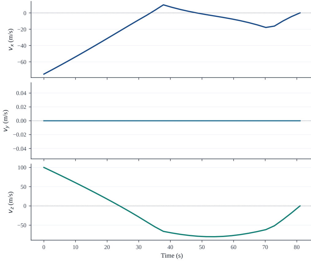
图 4 速度分量时间曲线。上: v_x ; 中: v_y ; 下: v_z 。
