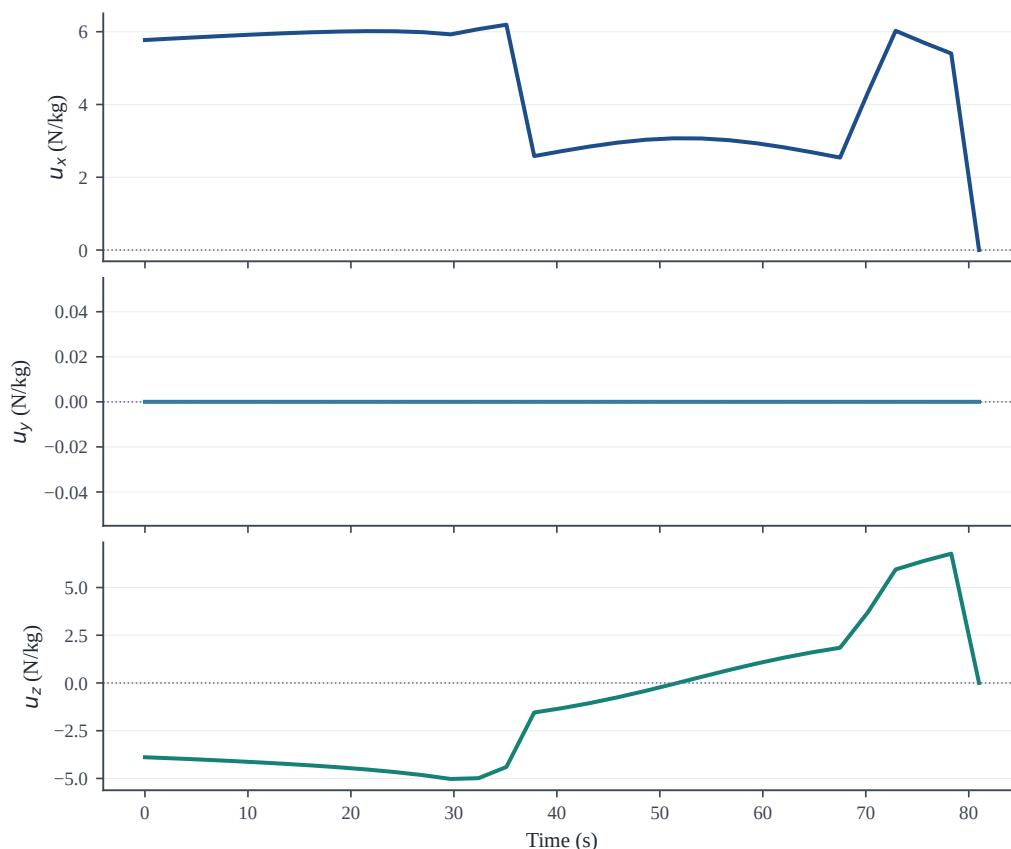
图 11 控制加速度分量 u_x, u_y, u_z 的时间演化曲线。
